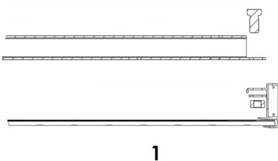
Abbildung 3: Detailansicht Backrail bzw. Modul (Schnitt) zur Montage der Backrails ( Ansicht von unten )
