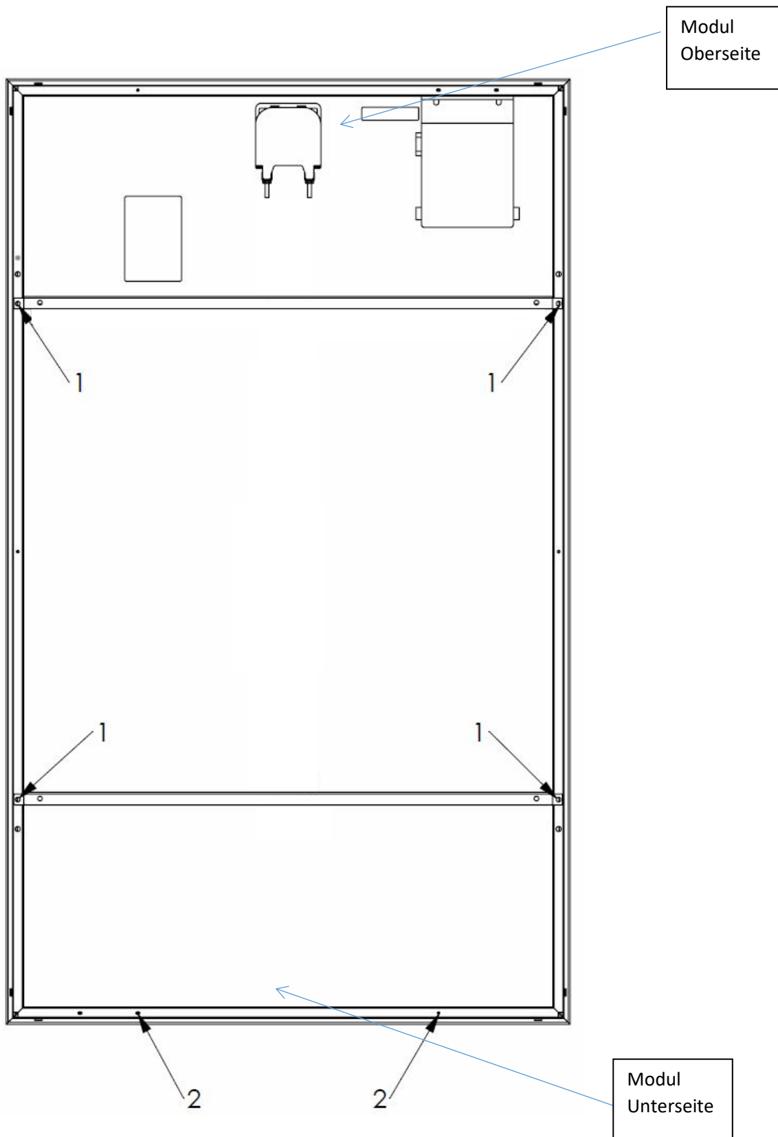
Abbildung 2: Schraubenpositionen zur Wandmontage
